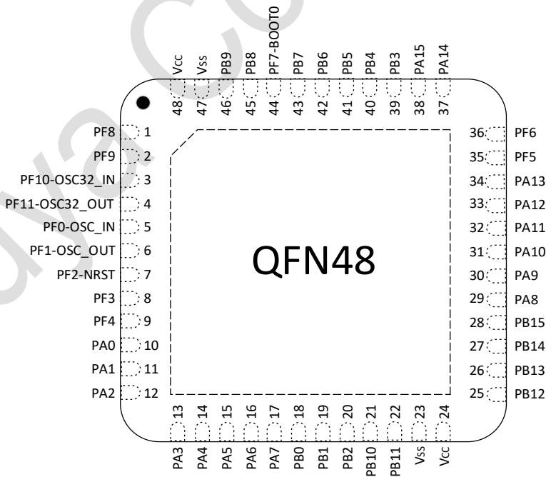
图 3-2 QFN48(6*6) Pinout1 PY32F031C1xU6 (Top view)
