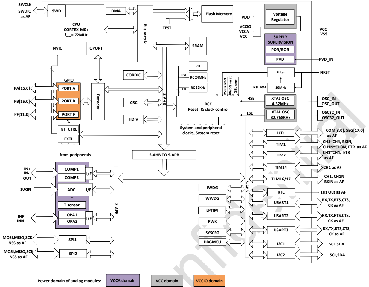
图 1-1 功能模块
